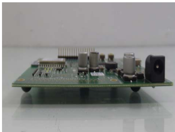
Figura 7 – Foto do ESE (parte lateral)
