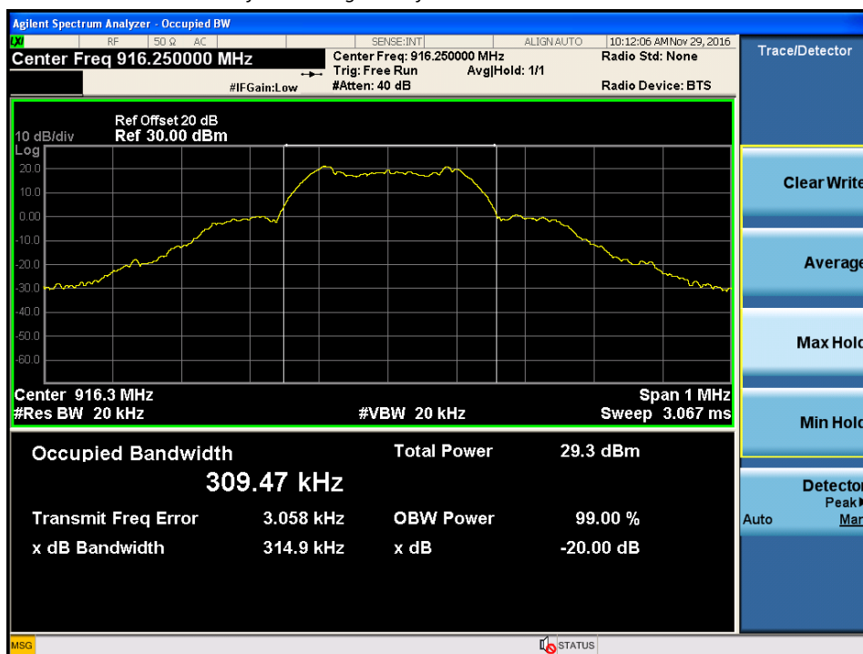
Gráfico 2 – Largura de faixa a 20 dB – Canal Central
