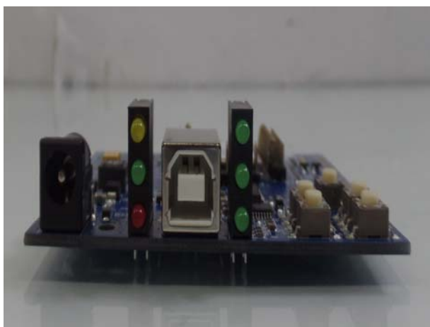
Figura 4 – Foto do ESE (parte inferior)
